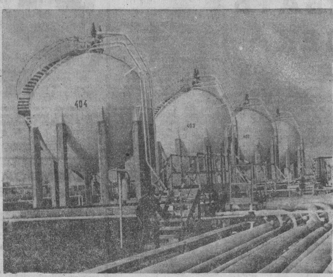
Вы видите на фотографии газохранилища, каждое вместимостью 400 кубометров. Это часть тех емкостей, в которые поступает природный газ, добываемый на Сегедских промыслах. Новый промышленный район успешно развивается и с каждым годом дает Венгрии все больше нефти и газа.
