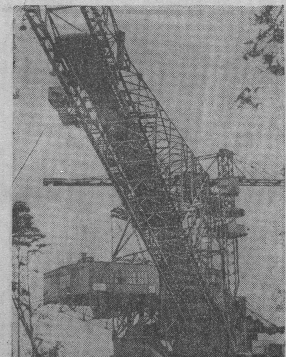
Высокопроизводительные механизмы для добычи угля открытым способом применяются в буровугольной промышленности Германской Демократической Республики. На этом снимке — мощный отвалобразователь типа «АС-1120» весом в 1.200 тонн и высотой в 38 метров, который будет использован на разработках комбината в Зенфенберге.
