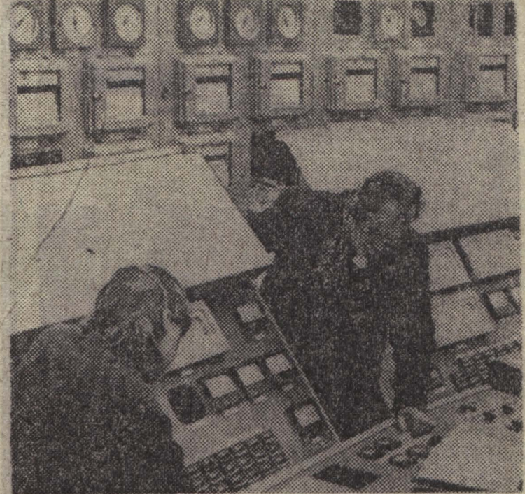
На три месяца раньше срока пущен восьмой энергоблок Литовской ГРЭС. Мощность электростанции достигла 1 миллиона 800 тысяч киловатт. Задание, поставленное в Директивах XXIV с'езда КПСС, выполнено. НА СНИМКЕ: пульт управления восьмого энергоблока.
