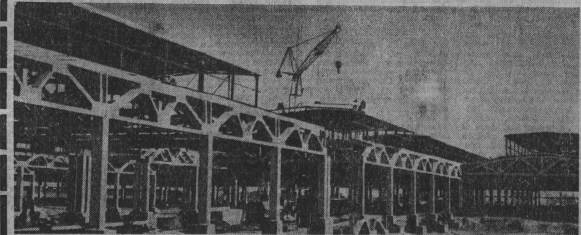
В Промышленновске сооружается фарфоро-фаянсовый завод. Сейчас строители возводят главный корпус. Монтаж ведет бригада С. З. Савькова из Кемеровского монтажного управления.
