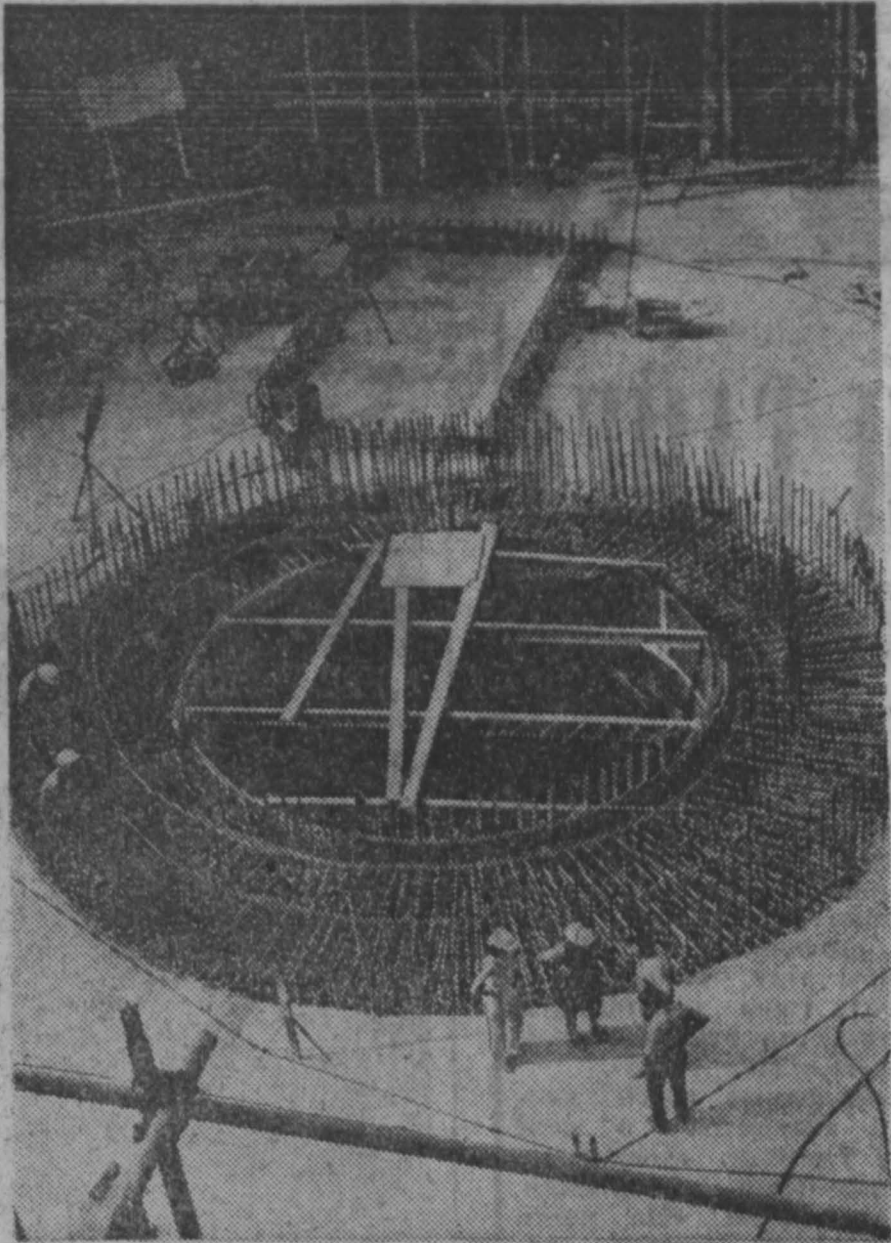
Строительство первой в Болгарии атомной электростанции в Козлодуже отмечено важным событием — началось возведение бетонных стен первого реакторного отделения, где разместятся один из реакторов станции мощностью 440 тысяч киловатт. Всего в Козлодуже будет установлено два таких реактора.
