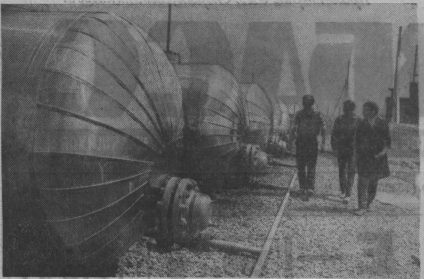
Оренбургская область. Инженеры, ученые и специалисты Всесоюзного научно-исследовательского института природных газов совместно с сотрудниками объединения Оренбурггазпром создали опытно-промышленную установку на скважине № 204 и работают над извлечением сероводорода из природного газа новым методом. Он позволит в короткие сроки получать очищенный газ, в котором нуждается народное хозяйство. Из удаленного же в процессе очистки сероводорода будет добываться сера для химической промышленности. НА СНИМКЕ: опытно-промышленная установка на скважине № 204. Фотохроника ТАСС.
