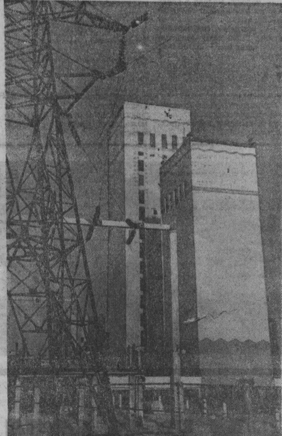
На реконструируемой шахте № 5-7 строители ведут последние монтажные и отделочные работы. Здесь впервые в Кузбассе вместо «бывших» металлических копров введены подпольные железобетонные. НА СНИМКЕ: башенные копры китевого и скипового стволов. Фото К. Николаева. г. Анжеро-Судженск.
