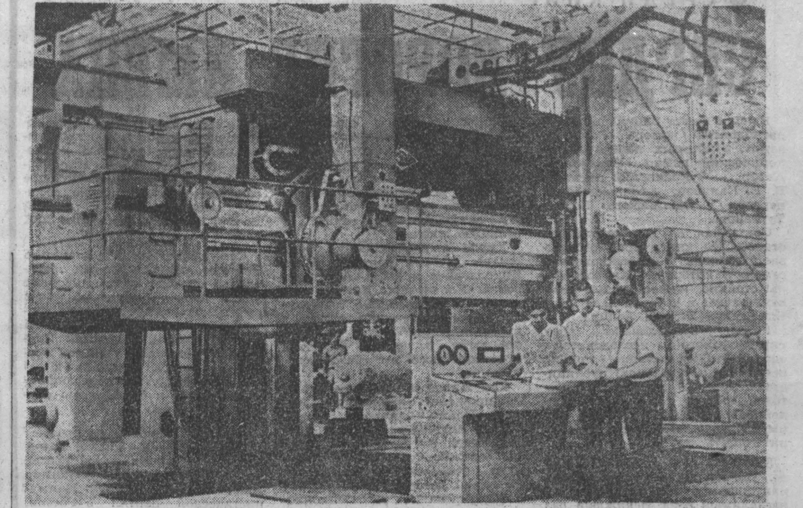
Индия. Общий вид одного из цехов завода тяжелого машиностроения в городе Ранчи (штат Бихар), построенного с помощью Советского Союза. Это предприятие выпускает оборудование для нефтяной, цементной и химической промышленности страны. Фото АДН—ТАСС.
