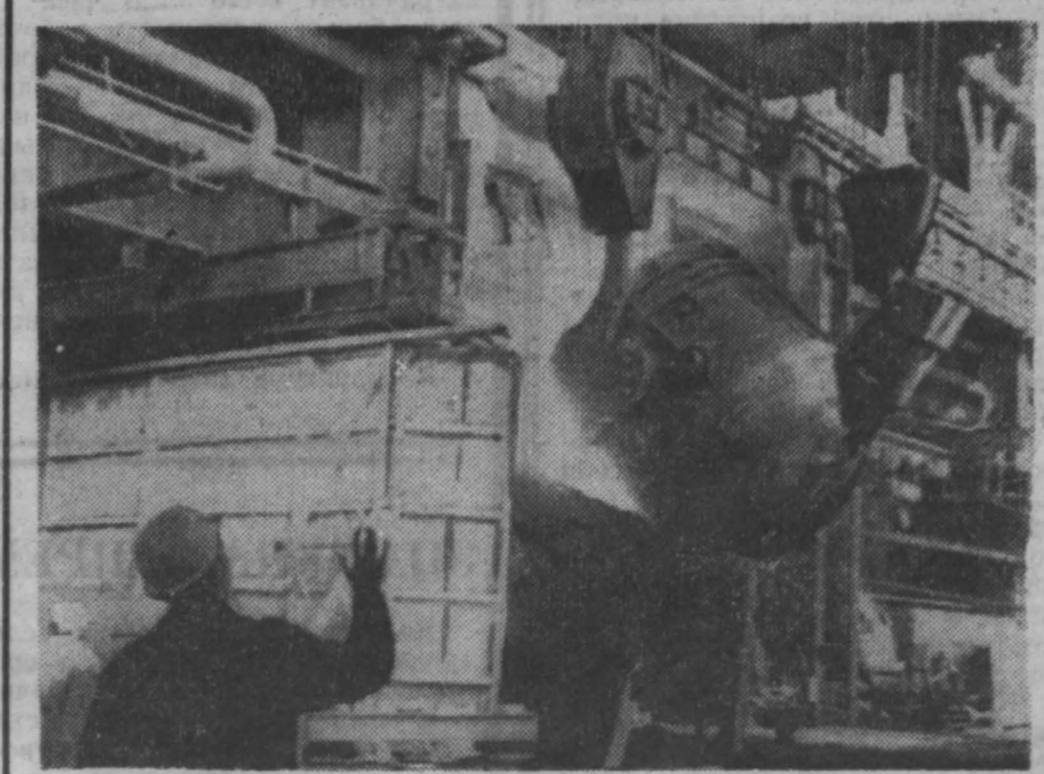
Отлично несут трудовую вахту конструкторы Зависба. Коллектив цеха в августе выдал несколько тысяч тонн серпильного металла. Одной из лучших считается смена Николая Пушицкого. НА СНИМКАХ: заливка чугуна в конвектор; мастер производства Н. С. Ткаченко и начальник смены Н. В. Пушицкий. Фото П. Костюкова.
