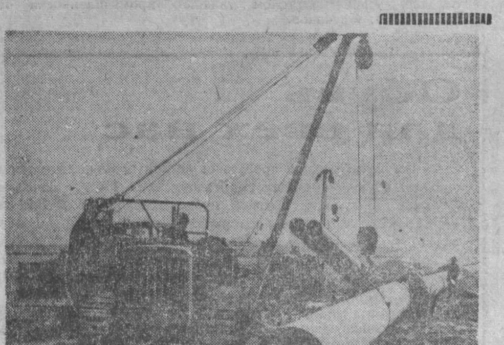
Началось строительство 350-километрового магистрального газопровода Душанбе—Яван. Уже в этом году природное топливо поступит к первому агрегату строящегося в Яванской долине мощной теплоэлектростанции. НА СНИМКЕ: монтаж газопровода Душанбе—Яван. Фотохроника ТАСС.
