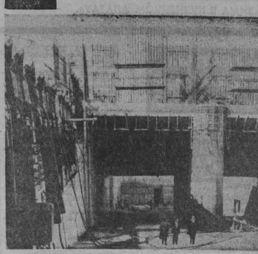
На Дунае в районе устья Джердап сооружается одна из крупнейших в мире гидроэлектростанций мощностью 2000 мегаватт и ежегодным производством 10,432 миллиона киловатт-часов электроэнергии. Также модернизируется судостроительная система, в результате чего пропускная способность в районе Джердапа возрастет в 4 раза. Строительство всего комплекса, которое осуществляется совместно на равных началах Югославией и Румынией, должно быть закончено в 1971 году.
