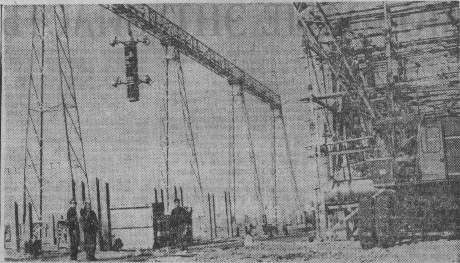
ОБЪЕДИНЕННАЯ АРАБСКАЯ РЕСПУБЛИКА. Каирская подстанция, расположенная неподалеку от египетской столицы, будет уникальным инженерным сооружением этого типа. Строительство находится на завершающем этапе. В этом году она будет сдана в эксплуатацию одновременно с 500-киловольтной линией электропередачи, которая через многие сотни километров свяжет Асуанскую ГЭС с Каиром.
