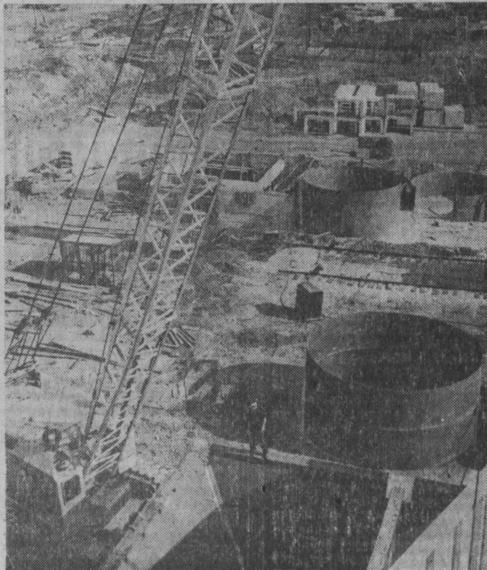
КУЙБЫШЕВСКАЯ ОБЛАСТЬ. На строительной площадке Волжского автомобильного завода работает несколько тысяч человек. Начато строительство главного корпуса вспомогательных цехов, бетонного завода, ТЭЦ и ряда других объектов. НА СНИМКЕ: вид одной из строительных площадок автозавода. ФОТОХРОНИКА ТАСС.
