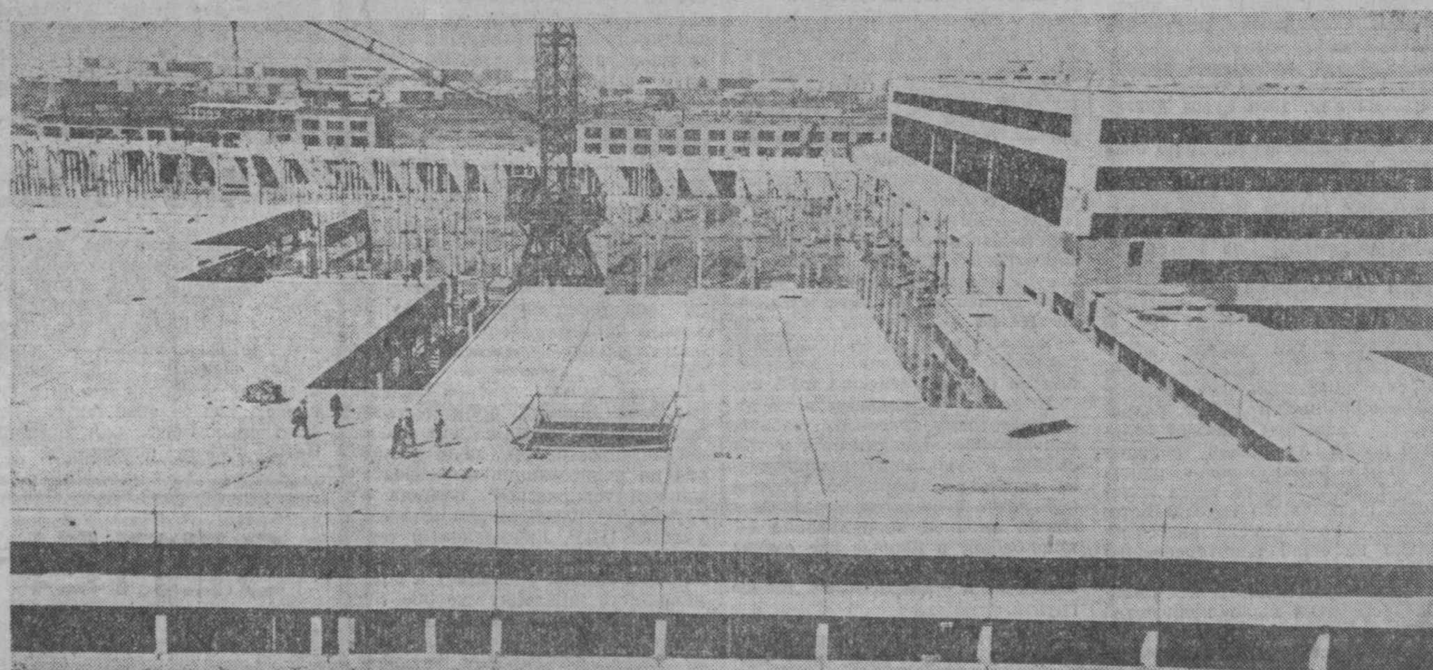
На окраине Кемерово идет сооружение завода химического волокна. Предприятие будет выпускать капрон и корд. В будущем году здесь вступит в строй опытная установка — завод в миниатюре. Она будет производить ежедневно 500 кг синтетического волокна.
