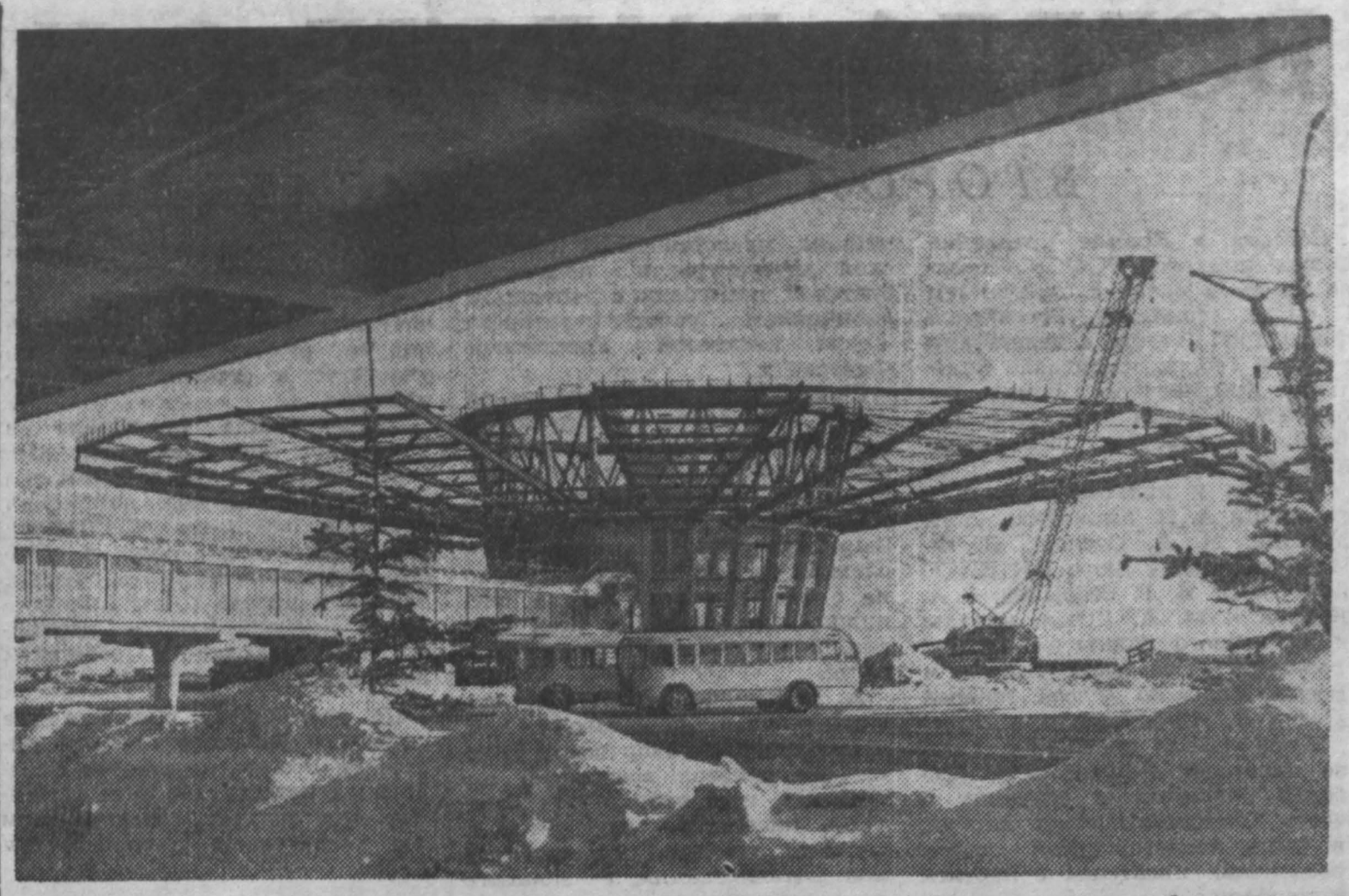
МОСКВА. В международном аэропорту Шереметьево строится посадочный павильон, который соединится с главным зданием аэровокзала стальной галереей. Круглая форма павильона позволит одновременно принимать и отправлять несколько самолетов. Пассажиры, прибывшие в Шереметьево, смогут перейти из самолета прямо в здание аэропорта.
