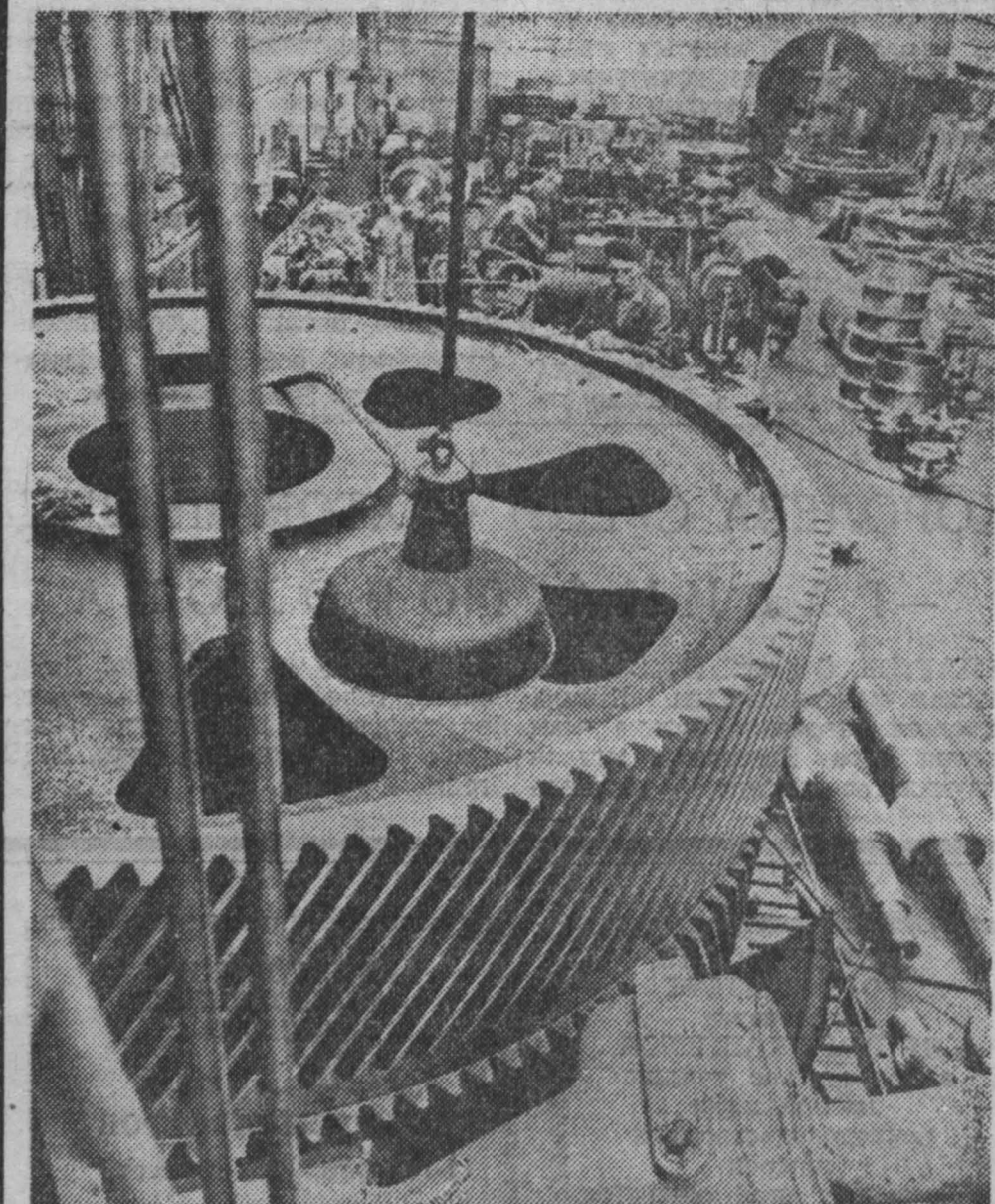
ЧССР, Западно-Чехия, на Пльзненском машиностроительном заводе имени В. И. Ленина изготовлено гигантское колесо для зубчатой передачи (его диаметр свыше четырех метров, вес — 50 тонн). Колесо является частью огромных ножей для резки стали.
