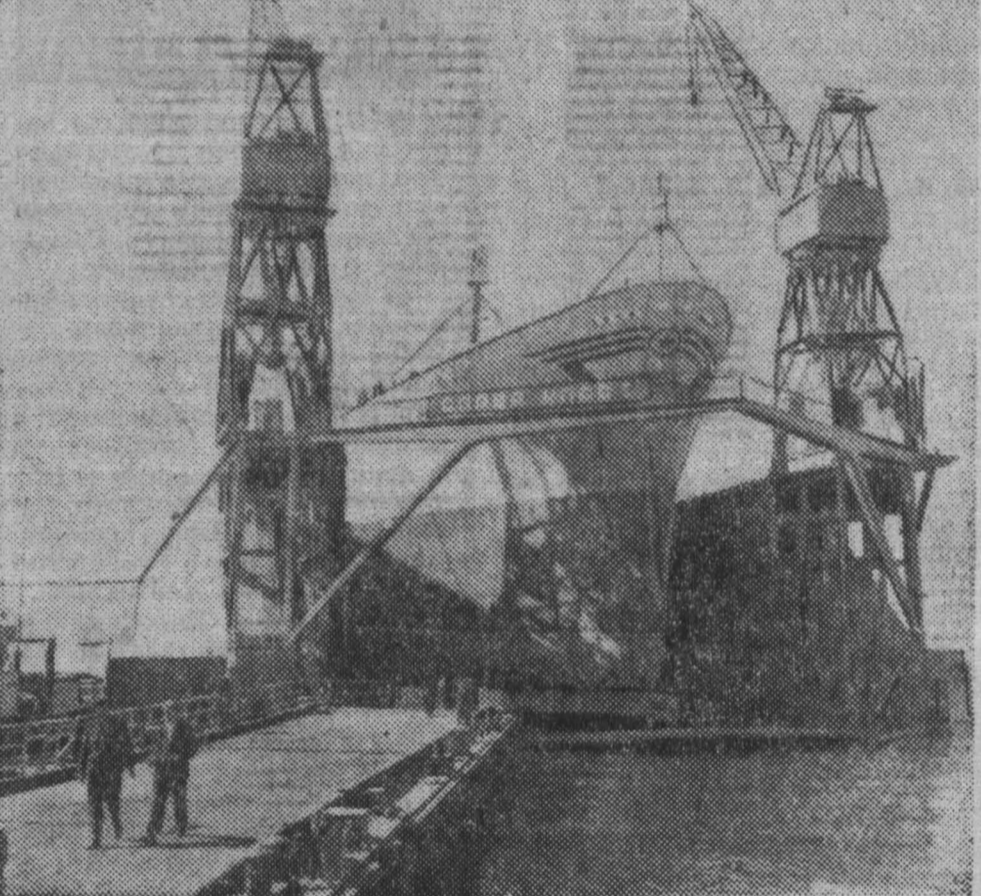
На Новороссийском судостроительном заводе вступил в строй металлургический плавающий док грузоподъемностью 27.000 тонн, длина его 217 метров. Док-гигант построен в Швеции на верфи «Геттаверкен» в Гетеборге. Фотохроника ТАСС.
