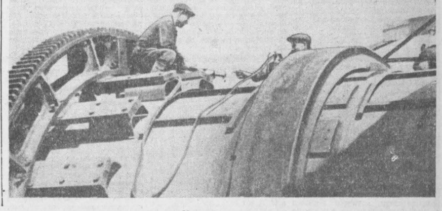
Накануне пуска в строй действующих — крупнейшая в Сусе Чернинская ЦОФ. Сейчас здесь производятся обкатка и доводка агрегатов, узлов. Новая фабрика будет обогащать 5 млн. тонн угля в год. На снимке: центровки сушильных барабанов производят слесари-монтажники И. Г. БЕДАРЕВ (справа) и А. Ф. КОРНЕВ. Фото А. Военкова.
