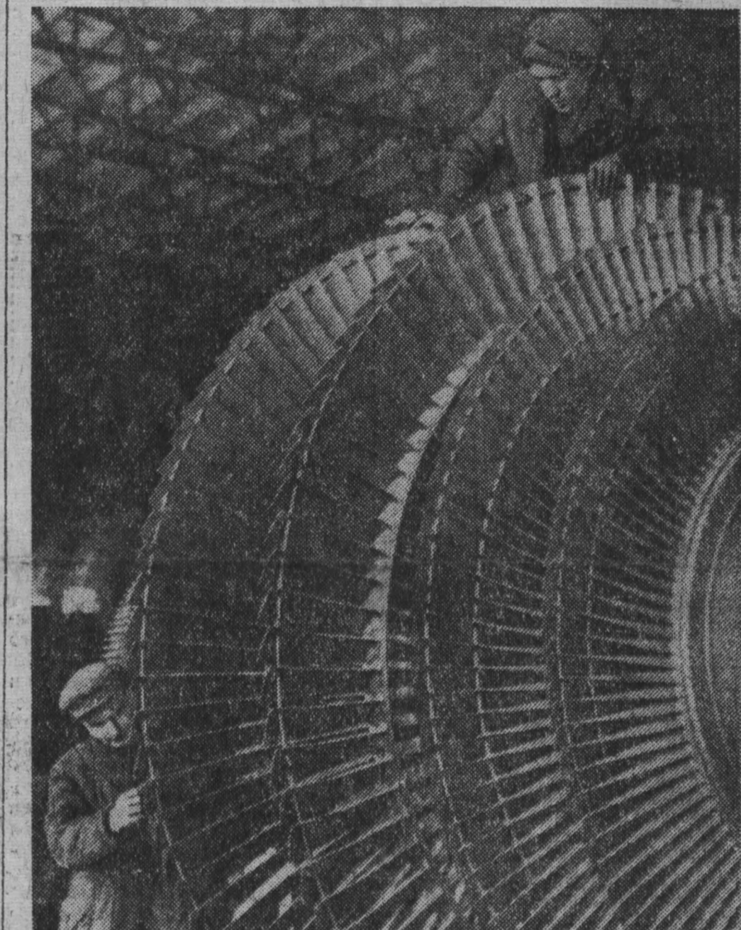
Большой самоотверженный труд вложен в строительство первой турбины Беловской ГРЭС. Имена членов бригады тт. Новикова и Попова навсегда войдут в историю сооружения одного из гигантов энергетической системы.
