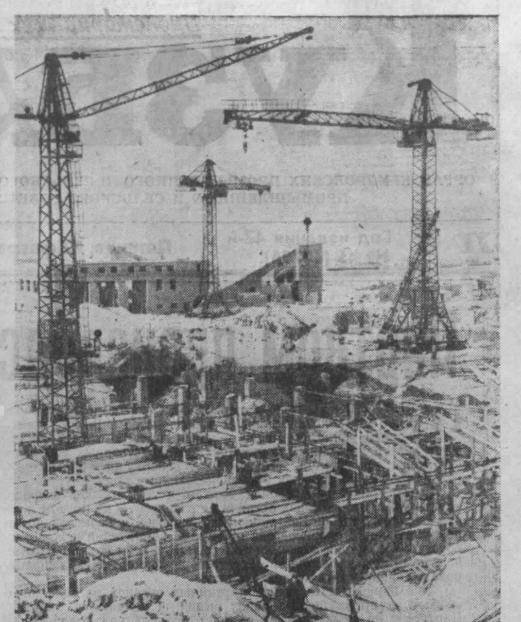
В полном разгаре сооружение Четтинской ЦОФ — одного из самых мощных и механизированных углеобогатительных предприятий нашей страны. Беловские строители спешат: фабрика крайне нужна шахтерам.
