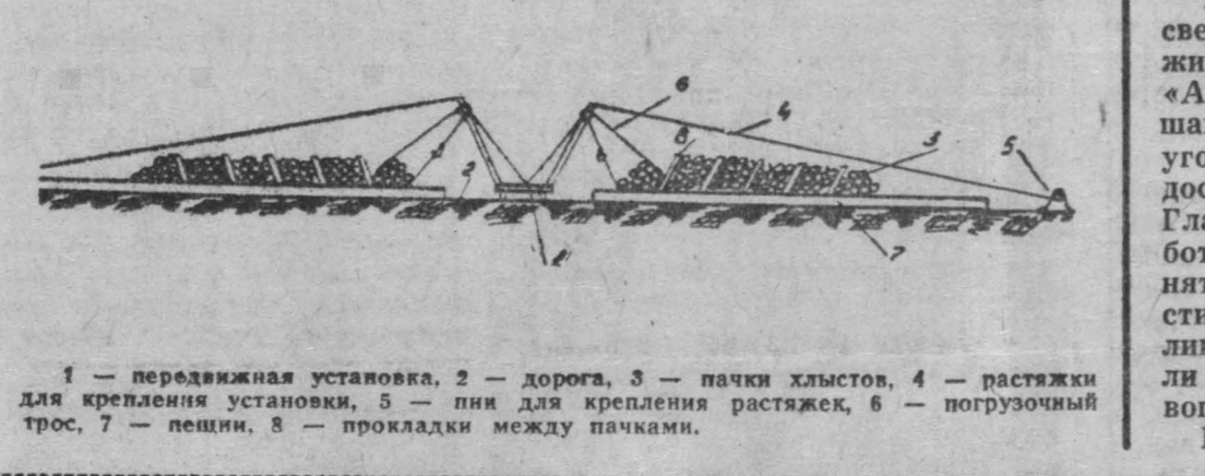
Рис. 3. 1 — передвижная установка, 2 — дорога, 3 — пачки хлыстов, 4 — растажи для крепления установки, 5 — пилы для крепления растяжек, 6 — погрузочный трос, 7 — лебедь, 8 — прокладки между пачками.
