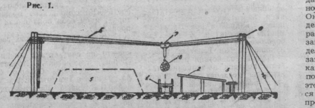
Рис. 1. 1 — автомашина, 2 — разделочная эстакада, 3 — транспортер, 4 — тросы кабель-крана, 5 — штабель запаса хлыстов, 6 — мачты кабель-крана, 7 — кабель-кран, 8 — разгруженные хлысты.
