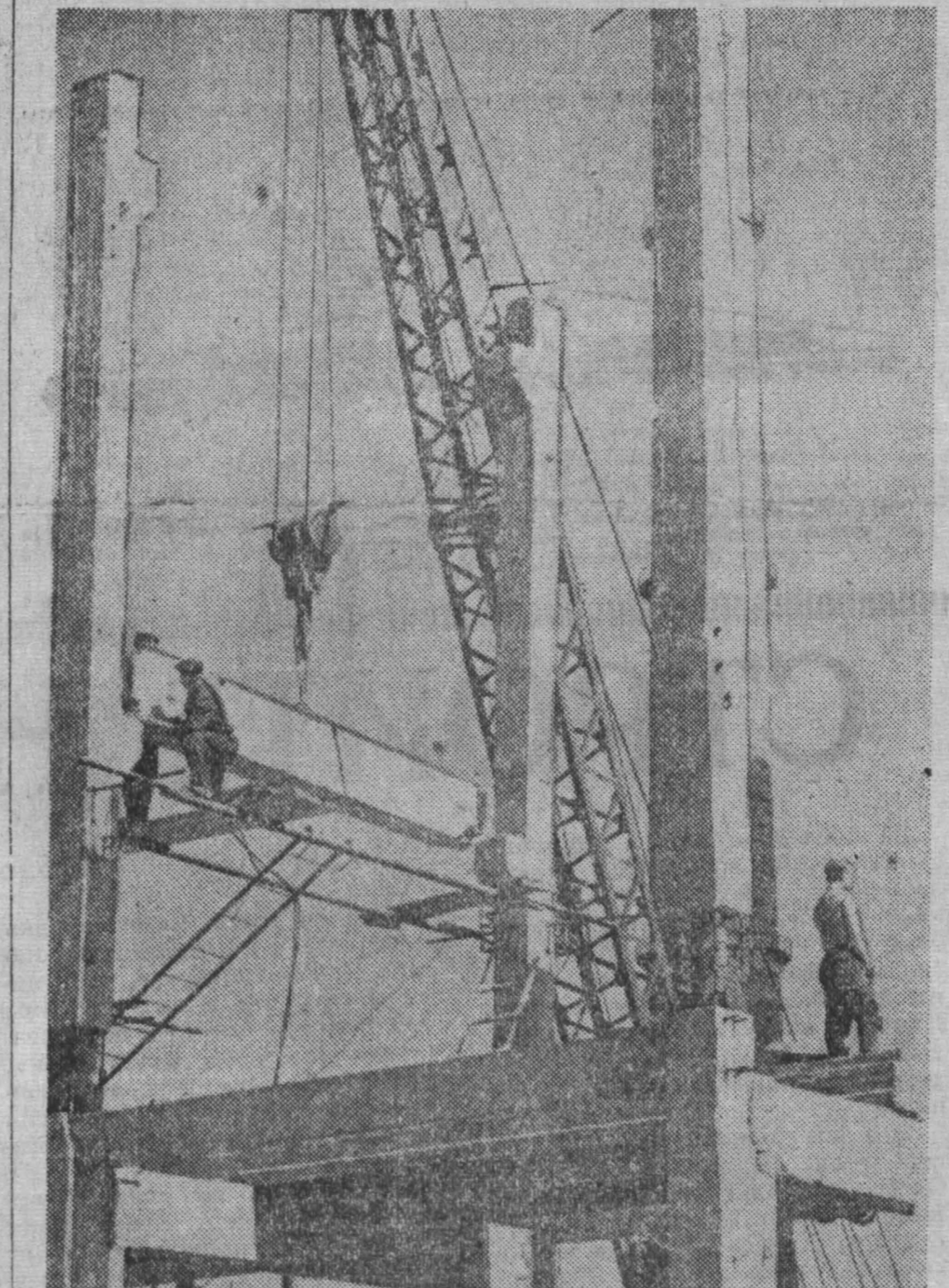
Общий вид сооружения пылепитателя котла Томь-Усинской ГРЭС. Фото В. Кафо.
