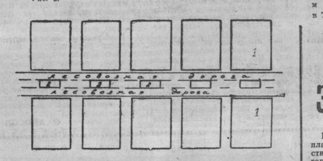
Рис. 2. 1 — штабеля хлыстов, 2 — места установки передвижной погрузочной мачты.
