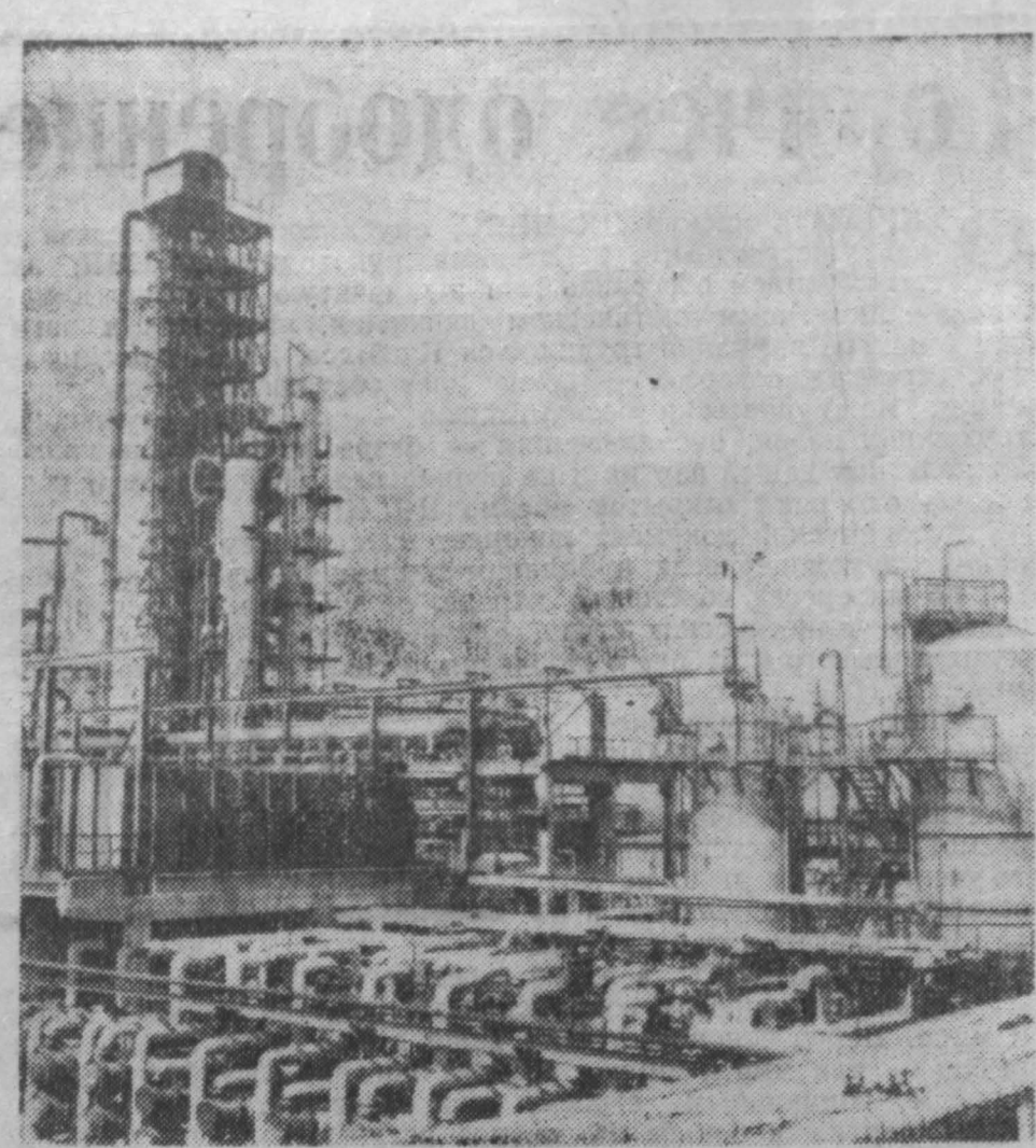
Растет большая химия нашей страны. В Белоруссии сдана в эксплуатацию первая технологическая линия. Полочного нефтеперерабатывающего завода. На снимке: вид атмосферно-вакуумной трубчатки. Фотохроника ТАСС.
