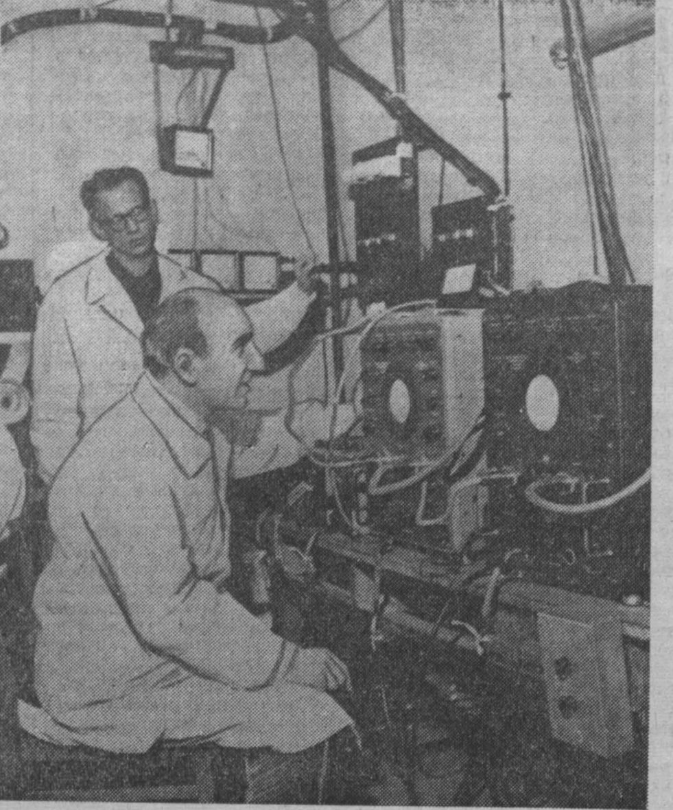
ПОЛЬСКАЯ НАРОДНАЯ РЕСПУБЛИКА. В лаборатории промышленной радиологии Варшавского института электротехники введен в действие первый польский бетатрон — прибор для ускорения электронов до больших энергий. Бетатрон имеет малые размеры.
