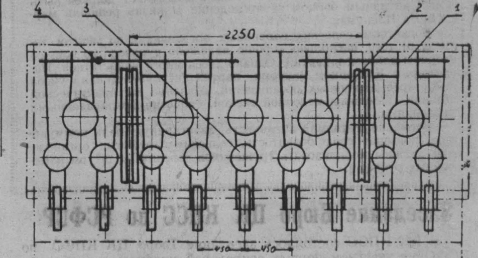
Рис. № 1. Схема расположения сошников и колес на междурядьях 45 см. 1 — трансмиссионный вал; 2 — туковывсевающий аппарат; 3 — высевающий аппарат; 4 — соединительная муфта удлиненного трансмиссионного вала.
