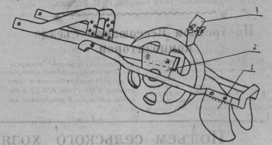
Рис. № 2. Переоборудованный прикатывающий каток. 1 — загорт; 2 — пластина; 3 — кронштейн части.
