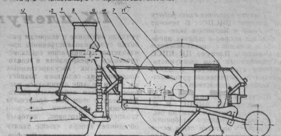
Рис. № 3. Схема установки на секции «СКГК-6В» приспособления для внесения удобрений одновременно с посевом сахарной свеклы. 1 — туковывсевающий аппарат; 2 — кронштейн; 3 — балка; 4 — поворотный сошник; 5 — кронштейн крепления сошника; 6 — туковывсевающий сошник; 7 — цепь; 8 — рычаг подема сошника; 9 — вал рычагов подема сошников; 10 — звездочка; 11 — тяга; 12 — средний угольный штифт.
