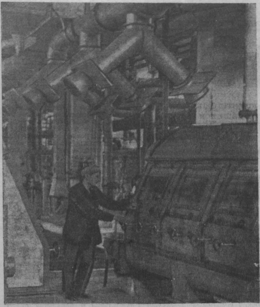
Кемеровский глинозёмбинат. Отсюда сейчас идет потребителям новая ценная продукция — лактам. Коллектив производств хлоролактама, готовясь достойно встретить 45-ю годовщину Великого Октября, неустанно совершенствует технологию, наращивает выпуск продукции.
