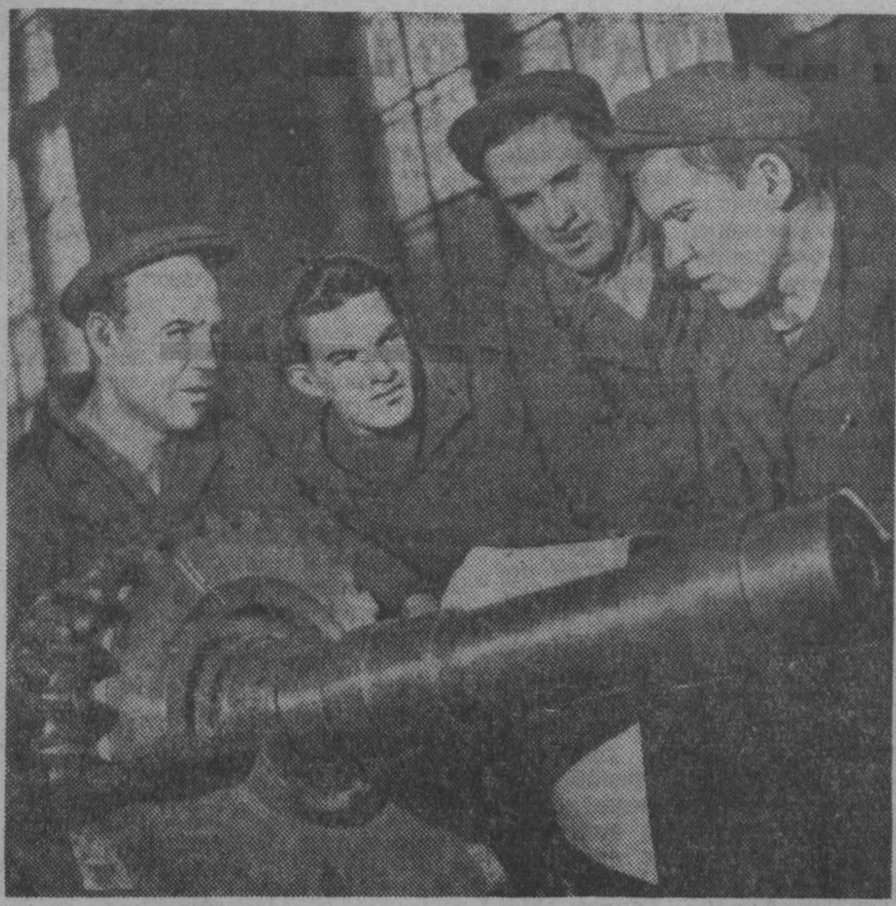
Хороший подарок Первому изготовителю бригады слесарей-сборщиков Николаю Кунцову с Прокопьевского механического завода. Она ведет сборку нового проходческого комбайна для восстанавливающейся конструкции проходки шахты «Зенковские уклон» И. Жулькина. НА СНИМКЕ: бригадыр Н. КУЗНЕЦОВ, слесари В. ДЕРБЕНЕВ, П. ДЕЧИК и мастер участка В. ЖУРАВЛЕВ сверлят узлы комбайна по схеме.
