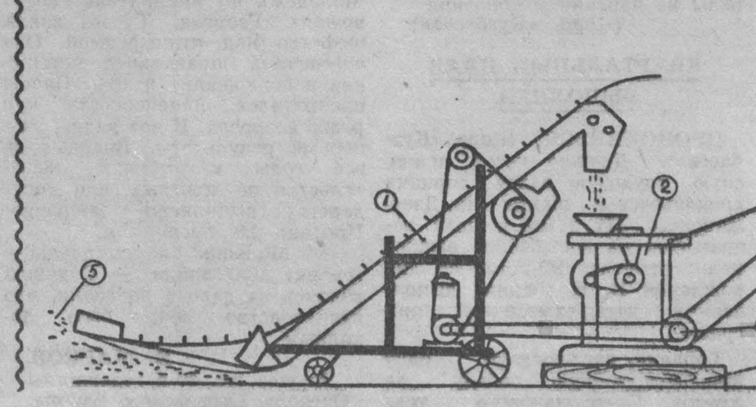
Инженер И. ЗЕЛЕНУХИН. Автоматическое приспособление (рис. № 2) для протравливания зерна с зернопогрузчиком, шнеком и элеватором.
