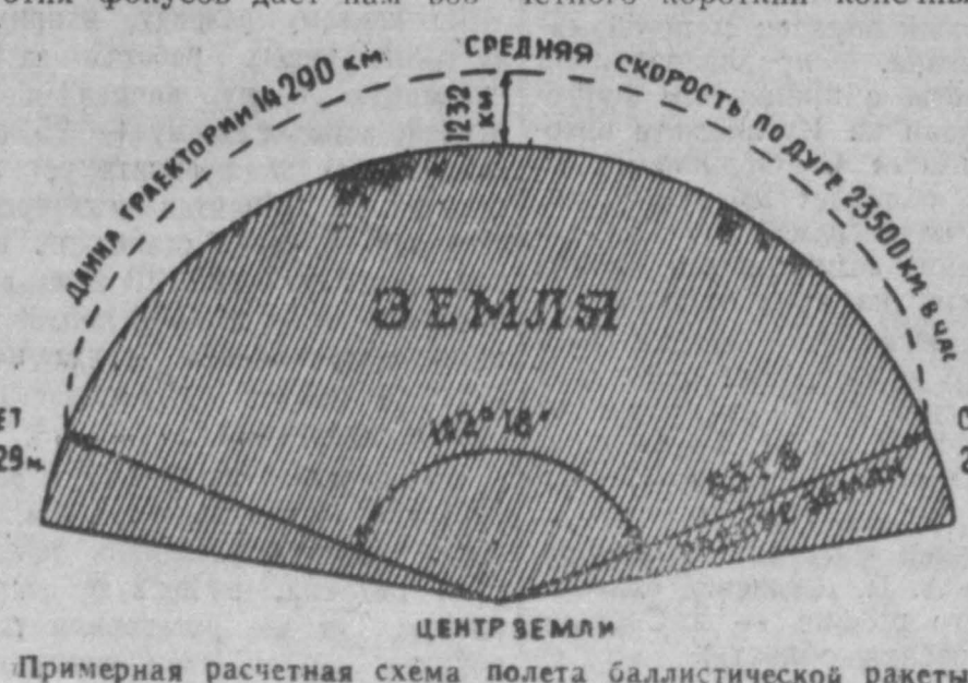
Примерная расчетная схема полета баллистической ракеты.
