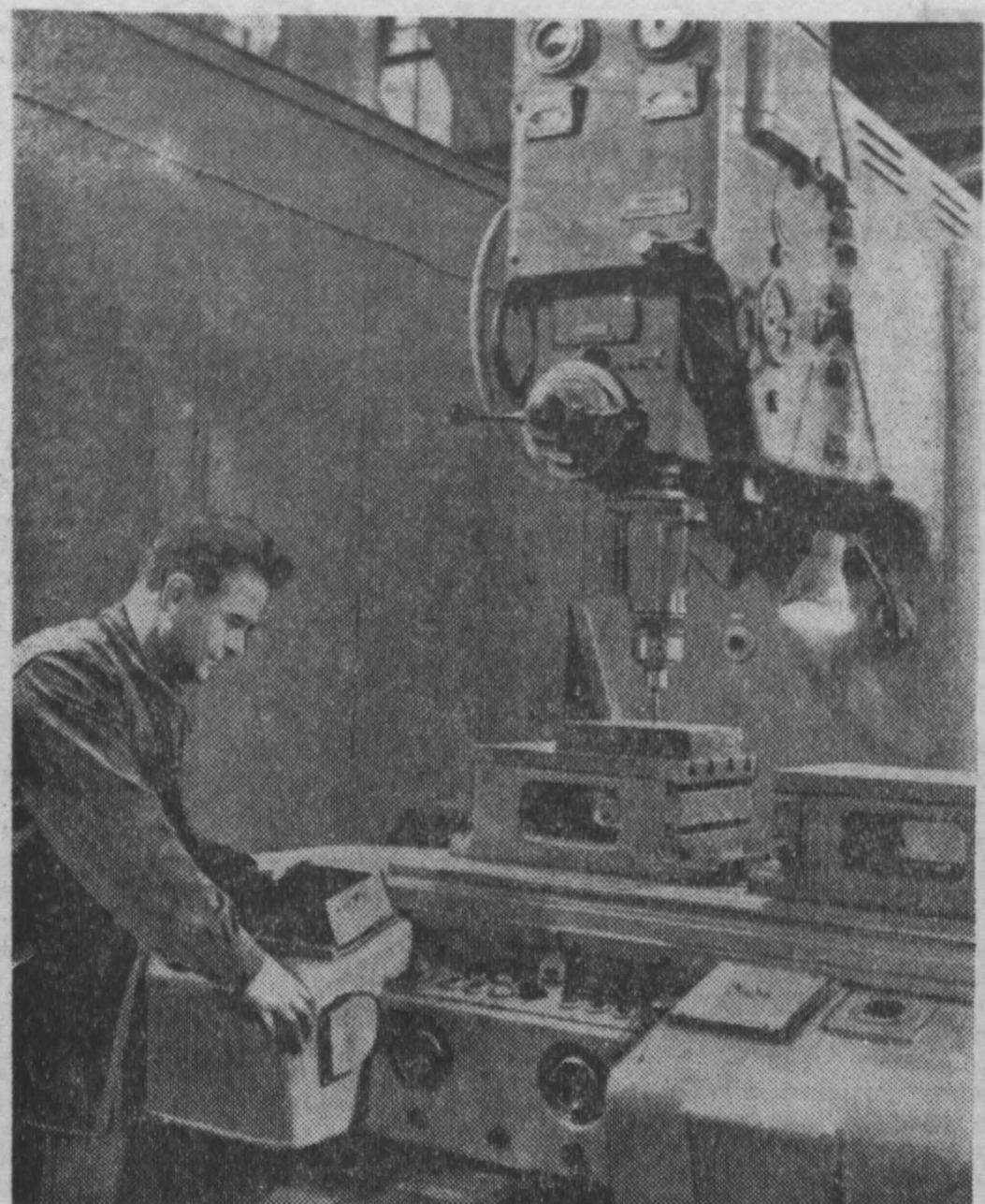
Коллектив завода координатно-расточных станков (Москва) создал первый в Советском Союзе координатно-расточный станок с программным управлением. Новый станок обладает точностью до 4 микронов. Он предназначен для инструментальной промышленности. Первый такой станок успешно прошел заводские испытания.
