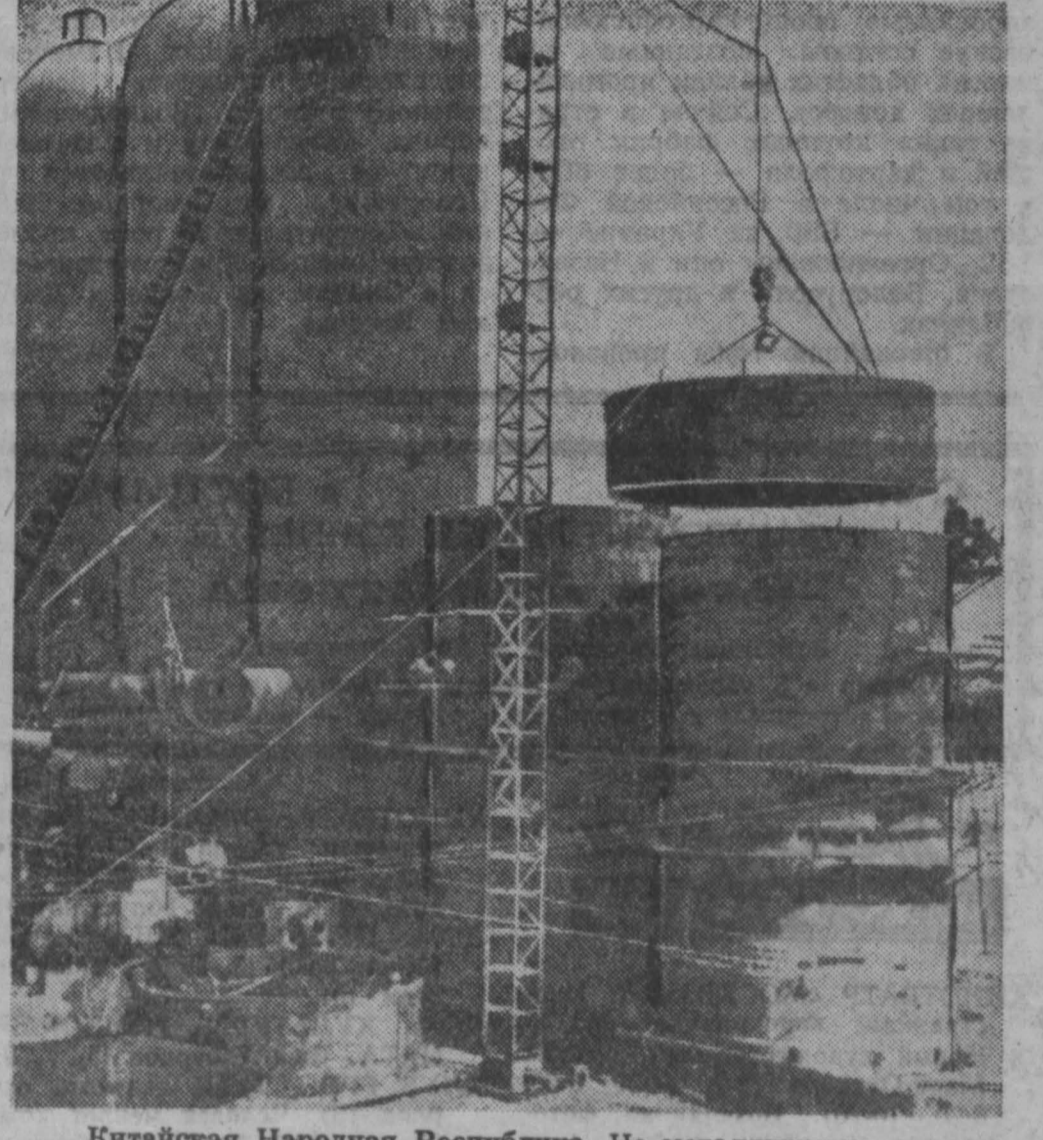
Китайская Народная Республика. На металлургическом заводе Ляочжоу (провинция Гуанси) строится вторая доменная печь. Первая доменная печь обьемом 255 кубических метров и стандартный завод уже даёт готовую продукцию. Все строительные работы будут закончены в 1963 году.
