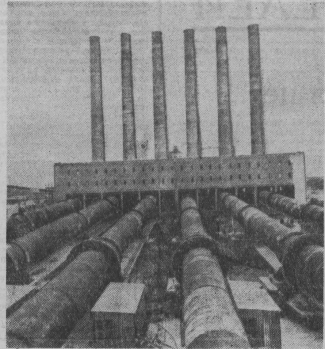
Польская Народная Республика. В Хелме сооружается крупнейший в стране цементный завод. Он вступит в строй в ближайшее время. Уже в этом году завод даст народному хозяйству страны около полумиллиона тонн цемента. НА СНИМКЕ: новый цементный завод. Фото Польского центрального фотоагентства.
