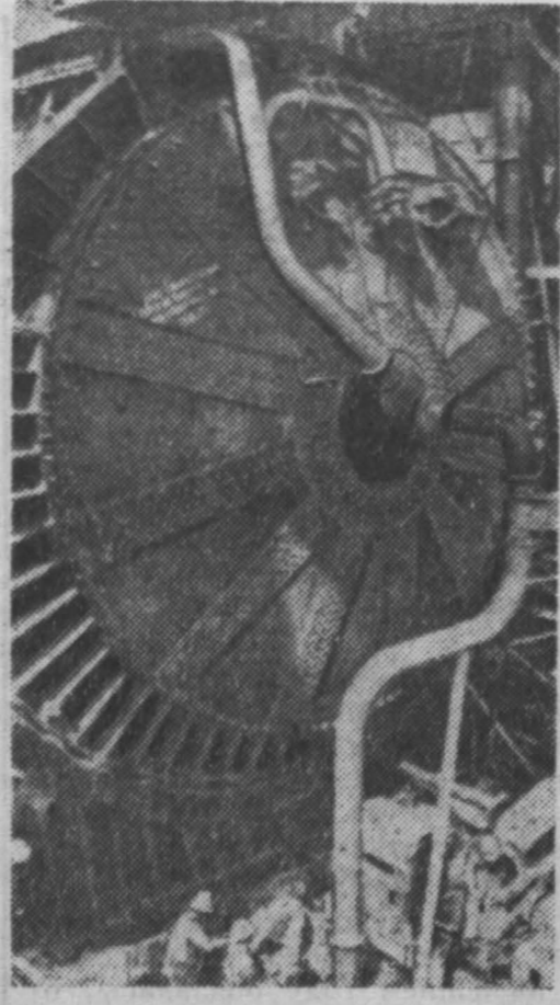
Китайская Народная Республика. Строители крупного металлургического центра в Батуте (Внутренняя Монголия) одержали новую трудовую победу. В рекордно короткий срок — за 15 дней закончена установка вращающейся печи.
