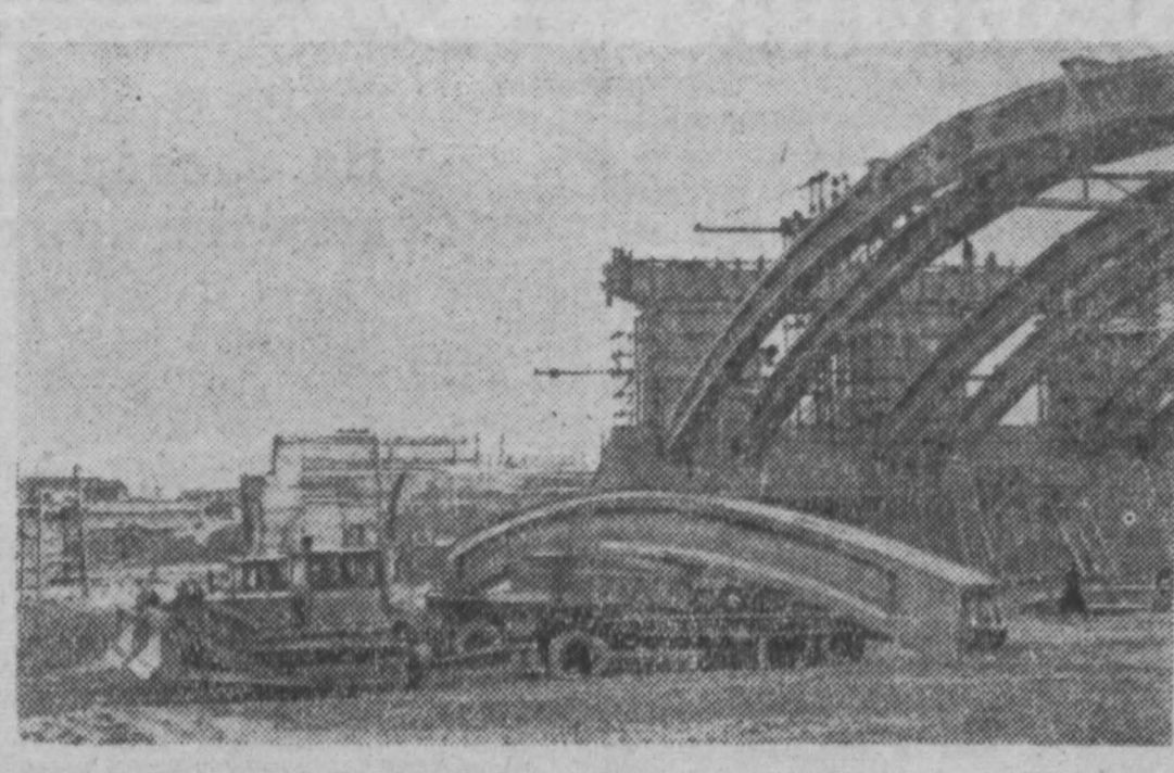
В Красноярске строится коммунальный мост через Енисей. Это будет уникальный по конструкции мост из сборного железобетона. Общая длина мостового перехода составит 2100 метров. НА СНИМКЕ: мощные бульдозеры доставляют пятидесятитонные попарки к месту установки их на опоры моста. Фотохроника ТАСС.
