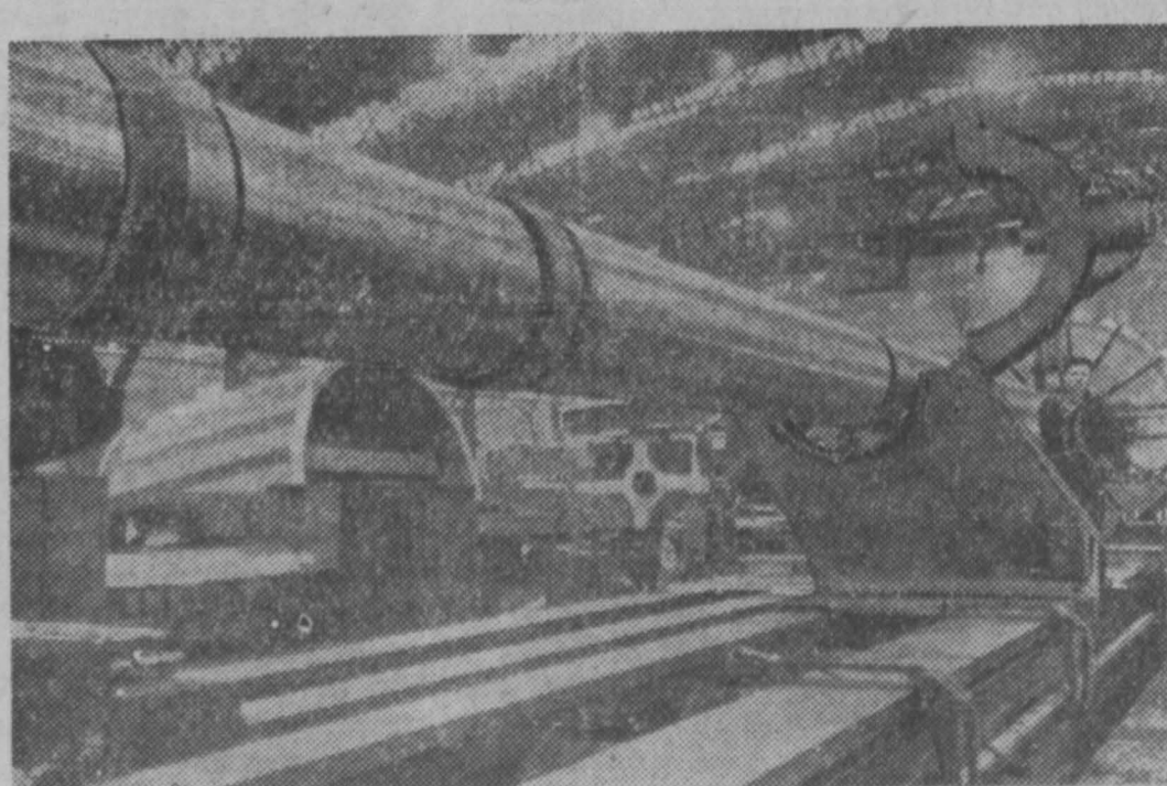
Свердловск. Уральский завод тяжелого машиностроения изготовляет коловный пресс с усилием 6 тысяч тонн. Общий вес всей установки 1.320 тонн. НА СНИМКЕ: обработка колонны пресса. Фотохроника ТАСС.
