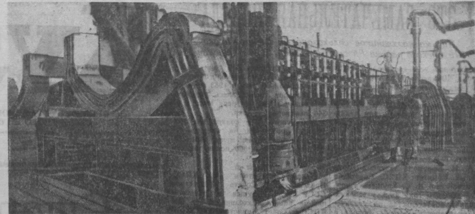
На Сталинском алюминиевом заводе сдачу в эксплуатацию новый электролизный цех. На снимке: новый электролизер.
