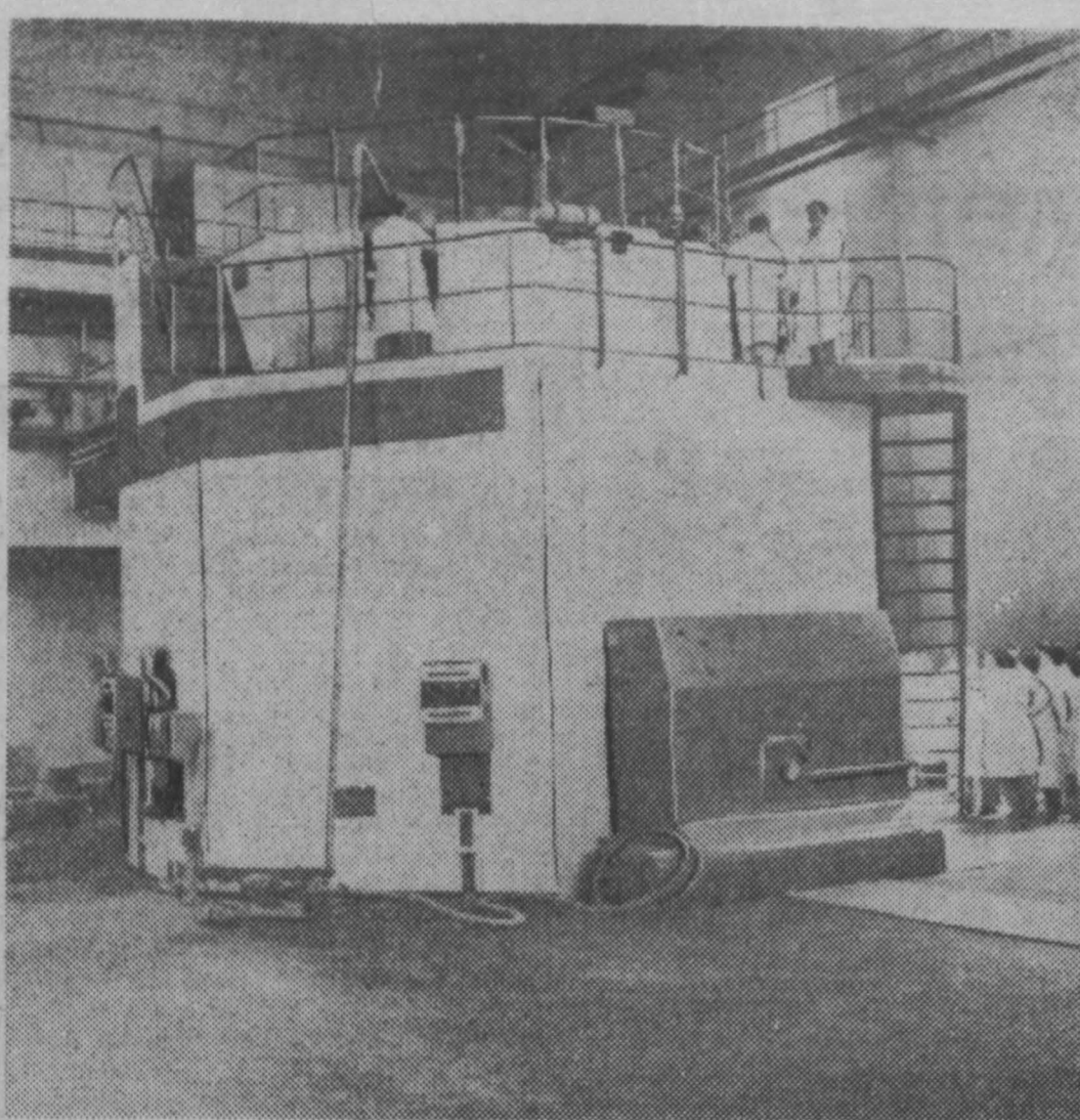
ТАШКЕНТ. В Институте ядерной физики Академии наук Узбекской ССР сдан в эксплуатацию атомный реактор, предназначенный для исследовательских целей.
