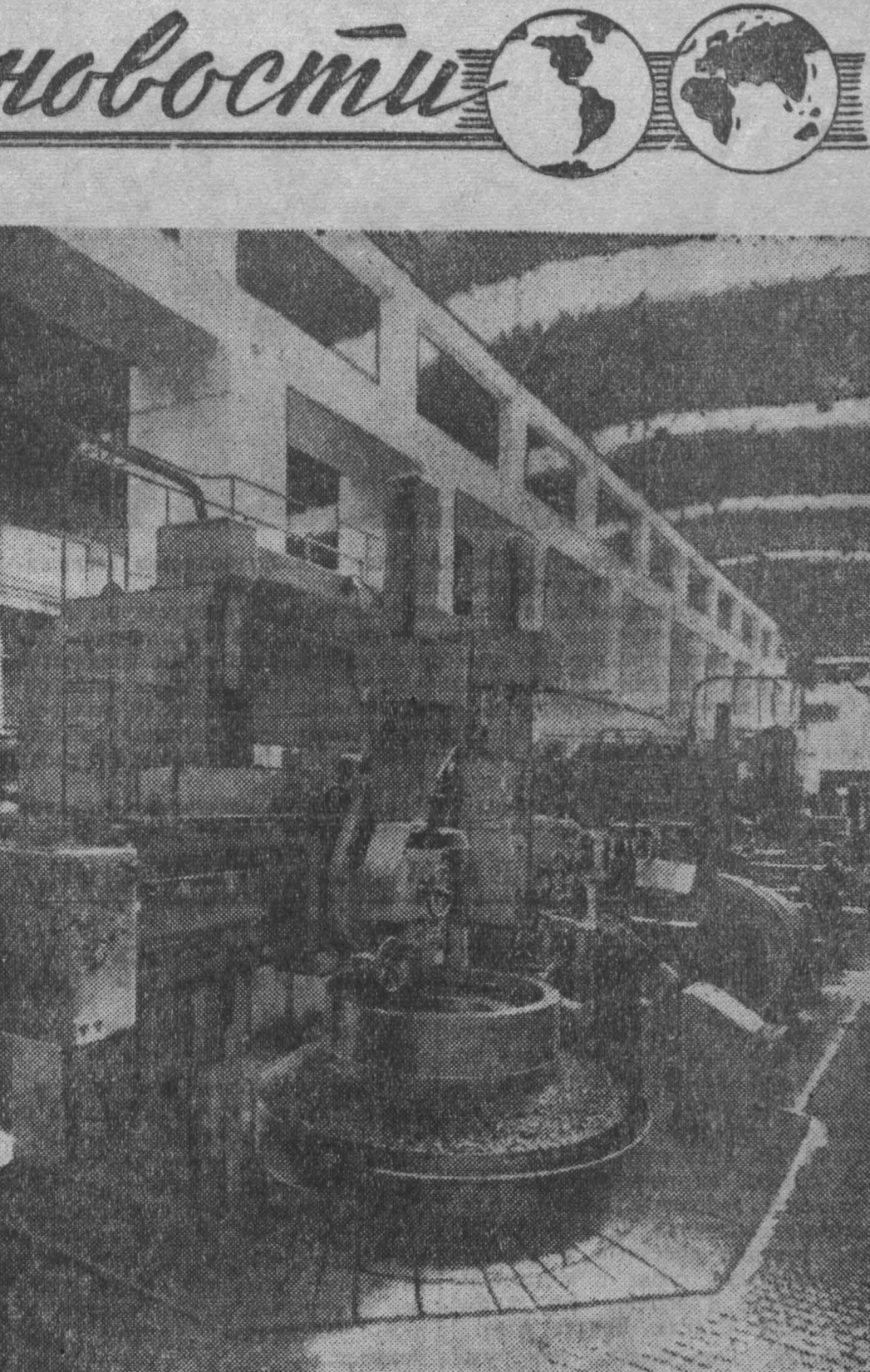
Машиностроительная промышленность Чехословацкой Республики увеличивает выпуск продукции по сравнению с довоенным уровнем в 5 раз. НА СНИМКЕ: в цехе машиностроительного завода имени Яна Швермы (город Брно). Токарь Ян Кайзер обрабатывает на карусельном токарном станке деталь пресса. Чехословацкое телеграфное агентство.
