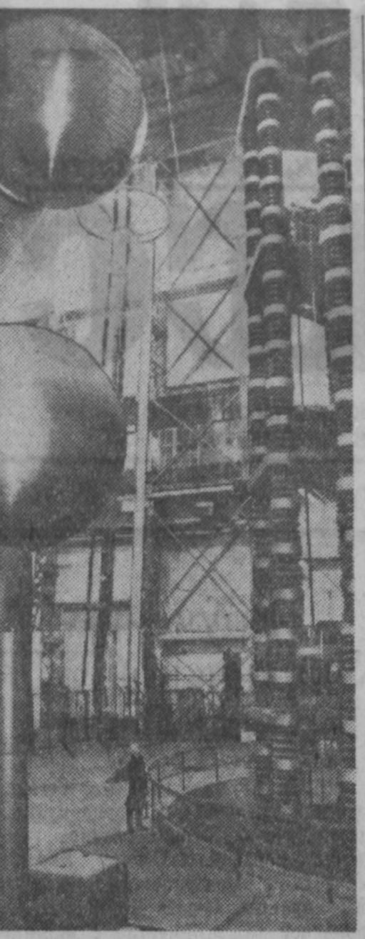
МОСКВА. Этот зал сооружен во Всесоюзном электротехническом институте имени Ленина для проведения испытаний трансформаторов и других электрических аппаратов высоких рабочих напряжений (до 330—500 тысяч вольт). Здесь уже установлен генератор импульсных напряжений на 7.200.000 вольт, идет монтаж каскада трансформаторов, предназначенных для испытания напряжений до 2.000.000 вольт, будет смонтирована установка для получения сверхвысоких напряжений постоянного тока.
