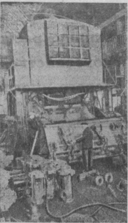
Эстонская ССР. На Таллинском машиностроительном заводе закончена сборка гигантского сланцевого комбайна, предназначенного для открытой добычи топлива. Длина машины около тридцати метров, ширина почти четыре метра. Добычу сланца комбайн производит полностью с помощью пневматических молотов, скрывающих отдельно сланца и породы. Благодаря этому топливо оказывается чистым и не требует дальнейшего обогащения. Двадцатитрёхметровый поворотный транспортер будет направлять сланец в автомосвалы или железнодорожные вагоны. Управлять комбайном будут всего два-три человека.
