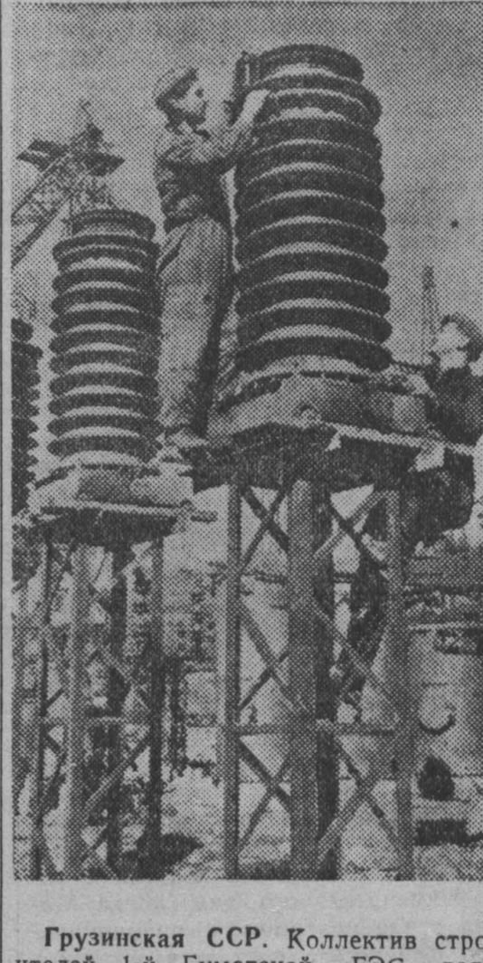
Грузинская ССР. Коллектив строителей 1-й Гуматской ГЭС взят обязательства сдать в эксплуатацию первые два агрегата к 7 ноября текущего года и остальные два — к концу декабря.
