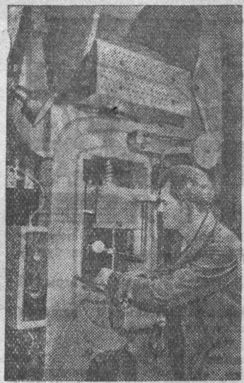
Москва. Производственный станок-конструкторный цех 3-го Государственного часового завода закончил сборку фрикционного прессы Д-278 мощностью в 25 тонн. Новые прессы найдут широкое применение в часовой, радиотехнической и приборостроительной промышленности.
