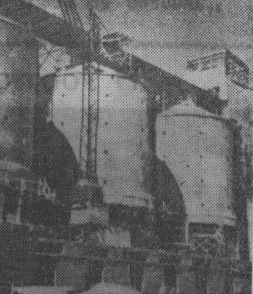
Польская Народная Республика. В конце прошлого года содовый завод в Янково выпустил первую продукцию. Сейчас предприятие ежедневно дает 300 тонн соды. В конце 1958 года будет производиться до 800 тонн кальцинированной соды ежедневно. В этих башнях хранится готовая для отправки продукция. Фотохроника ТАСС.
