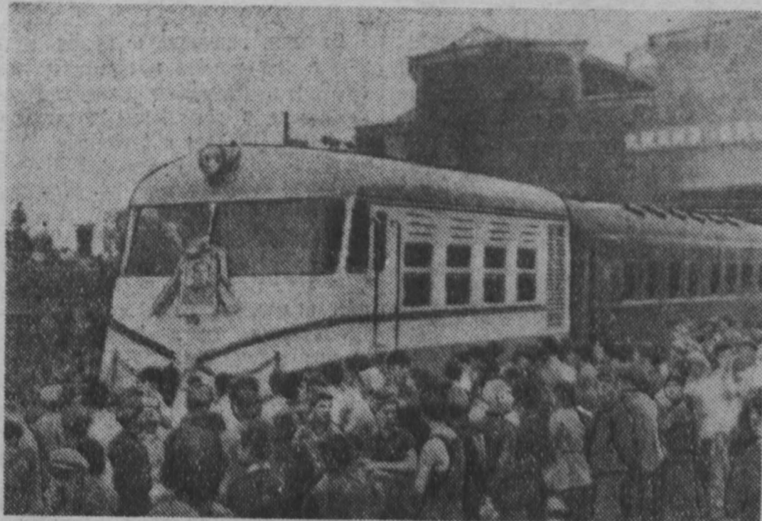
Китайская Народная Республика. Паровозостроители Чансиньдянского завода (близ Пекина) в честь первой годовщины образования КНР построили первый отечественный тепловоз. Все его оборудование создано на заводах Китая. Новый локомотив снабжен дизелем мощностью 600 лошадиных сил и может развивать скорость до 85 километров в час.
