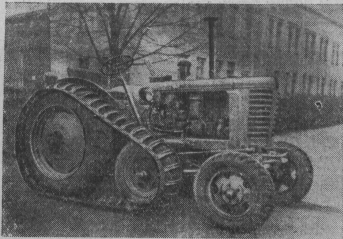
Минск. На тракторном заводе изготовлены экспериментальные образцы трактора «Беларусь» на полугусеничном ходу. НА СНИМКЕ: трактор «Беларусь» на полугусеничном ходу. Фотохроника ТАСС.
