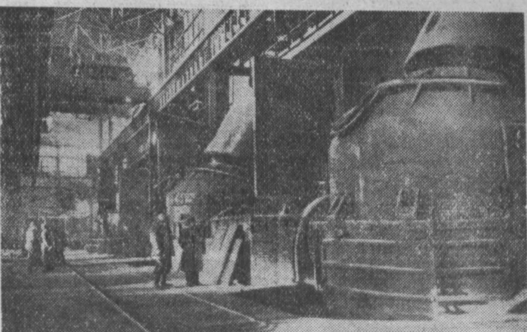
Днепропетровская область. На заводе «Криворожсталь» сдан в эксплуатацию конвертерный цех. Здесь начали производить сталь по новой технологии методом продувки чугуна технически чистым кислородом.
