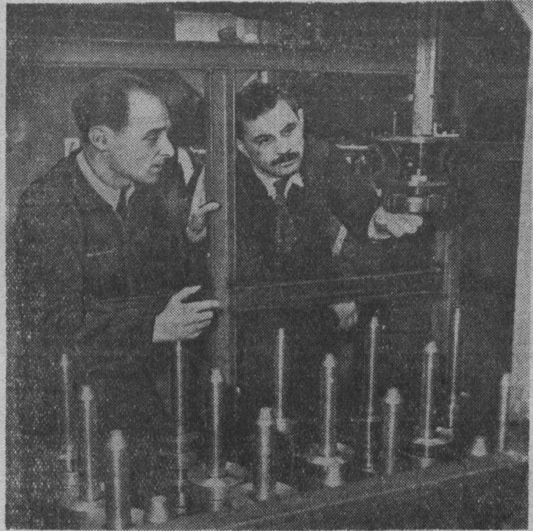
Москва. Коллектив научных сотрудников Экспериментального научно-исследовательского института металлорежущих станков в тесном сотрудничестве с работниками опытного завода «Станкоконструкция» создал новую автоматическую линию по изготовлению шестерен.
