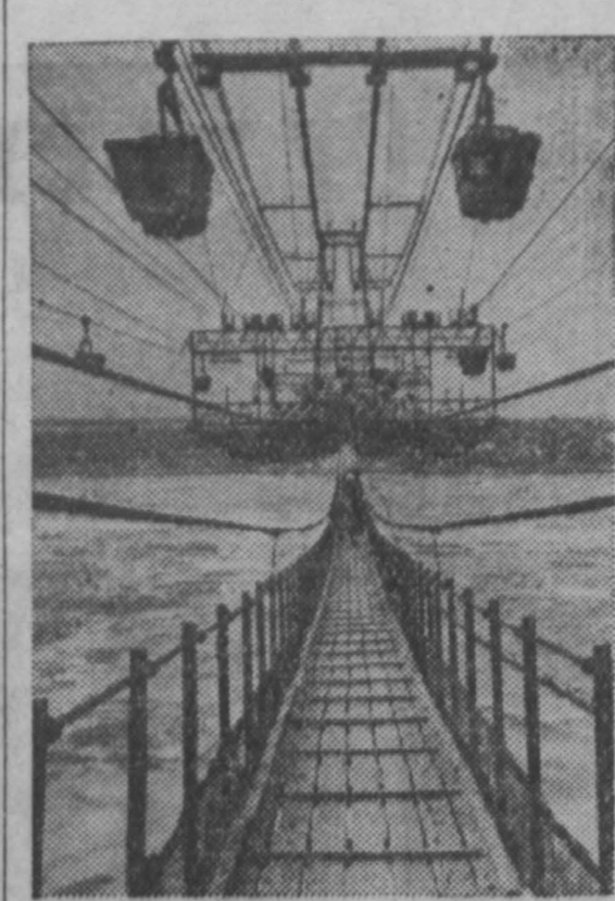
Строительство Сталинградской ГЭС. По подвесной канатной дороге через Волгу доставляется много строительных материалов с правого берега. Во время ледохода пешеходная подвесная дорога является единственным путем, по которому рабочие, живущие на правом берегу, могут попасть на левый.
