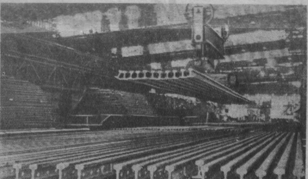
НА СНИМКАХ: подача стальных слитков из нагревательных колодцев на рольганг блуминга. Штабелевка готовых рельсов с помощью электро-Фото П. Костякова.
