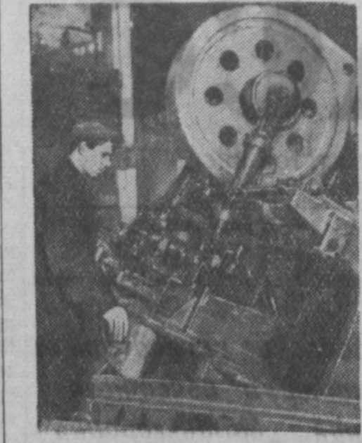
Горький. В арматурном цехе автозавода сконструированы и изготовлены первые два прессы-автомата для штамповки мелких автомобильных деталей из листового металла. Полосы металла захватываются специальными прессами и автоматически подносятся в штамповочный станок. Каждый пресс-автомат может выдавать за смену до 90 тысяч деталей и заменять шесть прессов с ручным податком.
