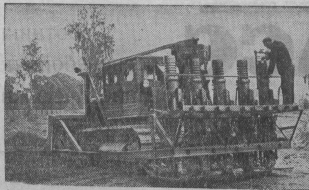
Латвийская ССР. На Рижском ремонтно-механическом заводе закончен монтаж новой дизельной трамбовочной машины для уплотнения грунта железнодорожного полотна. Машина смонтирована на тракторе «С-80». Глубина уплотнения вновь отсыпанного грунта полтора метра, ширина — три метра, производительность машины 450 кубических метров в час.
