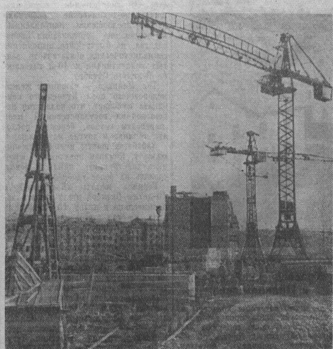
Строительство жилых домов для металлургов Кузнецкого комбината на проспекте имени Курако в городе Сталинске. Фото В. Скоробогатова.
