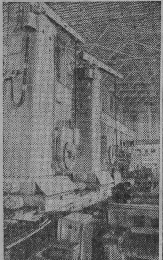
НА СНИМКЕ: агрегат из двух горизонтально-расточных станков. Фотохроника ТАСС.
