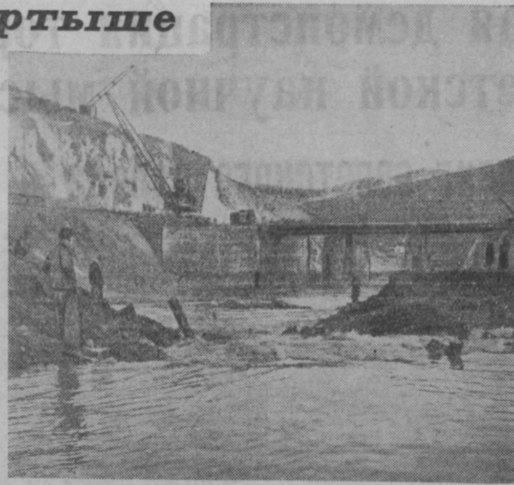
Строители Бухтарминской ГЭС одержали большую трудовую победу: в котловане первой очереди закончены работы по сооружению подводной части возвышенной плотины. 28 сентября 1957 года правобережный котлован был затоплен.
