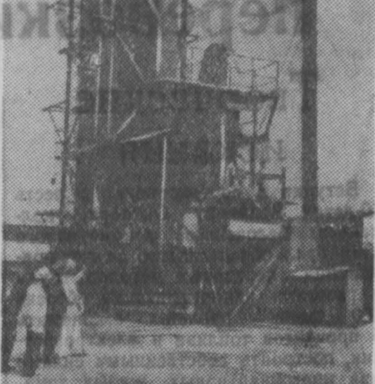
Минск. В Институте энергетической Академии наук Белорусской ССР разработан новый метод сушки зерна, основанный на чередовании процессов нагрева и охлаждения. Нагрев зерна производится в потоке горячих газов и протекает 4-5 секунд, т. е. в сотни раз быстрее по сравнению с существующими методами сушки зерна. После каждого прогресса — зерно подвергается охлаждению в потоке холодного воздуха. Все эти процессы происходят в специальной пневмогазовой сушилке, созданной сотрудниками института. Такие установки уже имеются в колхозе имени Ленина, Минском районе, и на минской базе «Заготзерно». Проведенные здесь опыты показали, что семенное зерно, просушенное через пневмогазовую сушилку, дает прибавку урожая на 10-15 процентов и выше.
